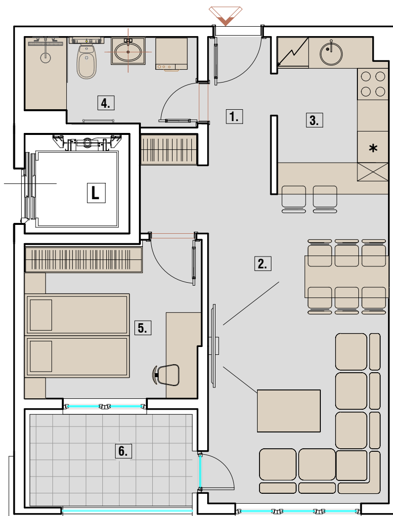
OSNOVA STANA
